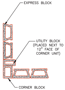
EXPRESS ODD CORNER DETAIL N.T.S.
