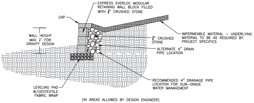
EXPRESS GRAVITY WALL DESIGN N.T.S.
