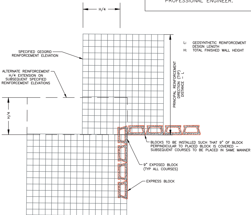
EXPRESS ODD CORNER DETAIL N.T.S.
