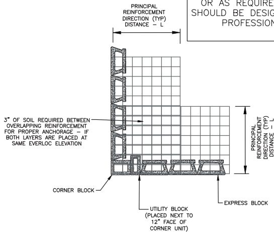
EXPRESS GEOGRID CORNER DETAIL N.T.S.
