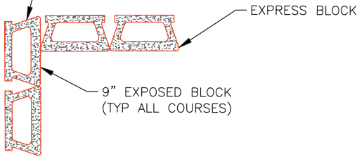
EXPRESS ODD CORNER DETAIL N.T.S.
